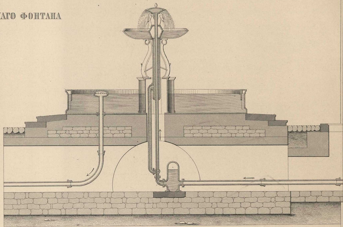
РАЗРѢЗЪ
